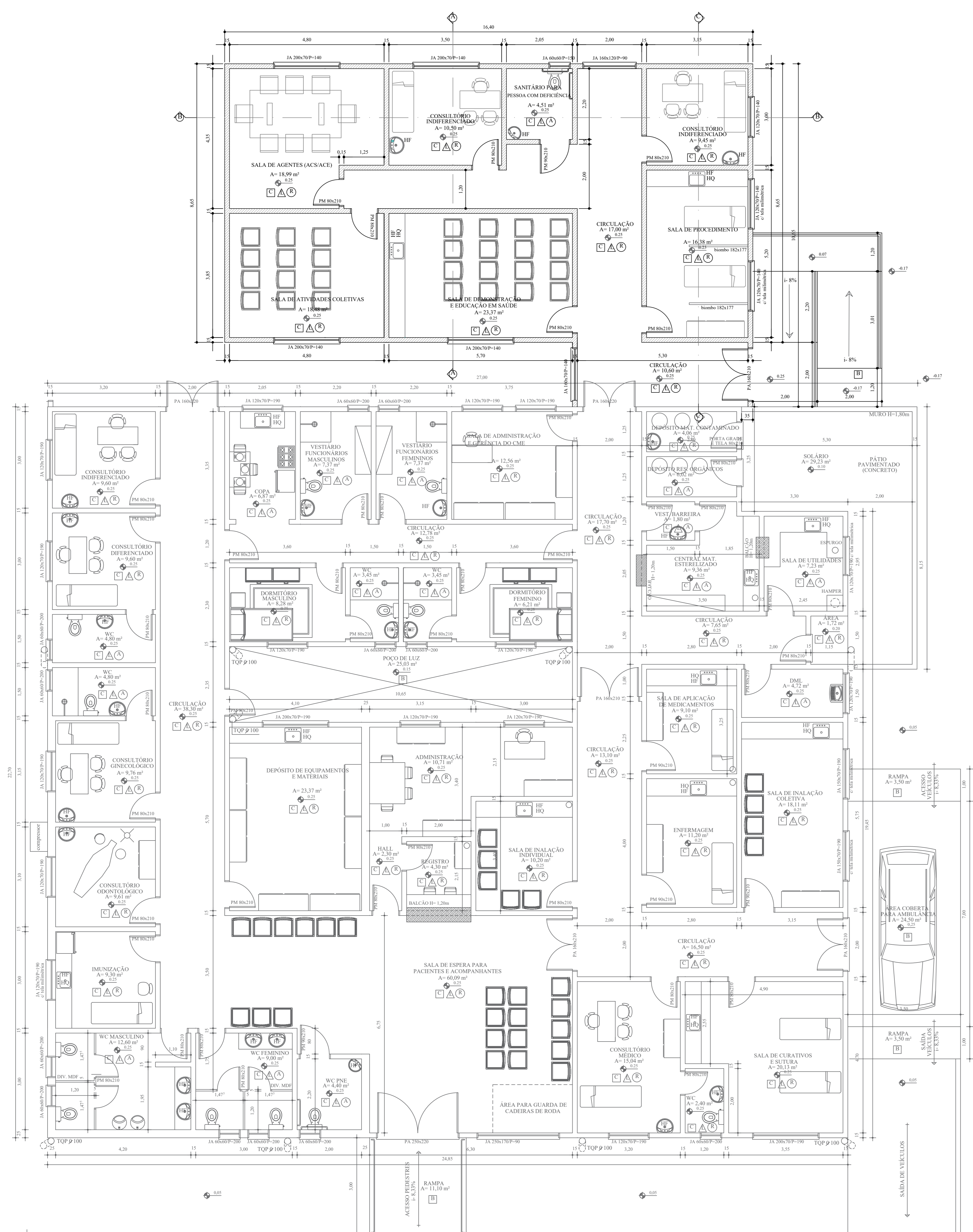
PLANTA BAIXA A= 717,00 m 2
